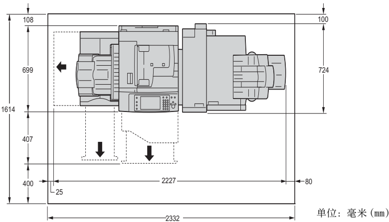
装有完成装订部 C3（小册子装订）（选装）、CD1 折叠组件（选装）、侧接收盘（选装）和大容量纸盘 B1（选装）时
