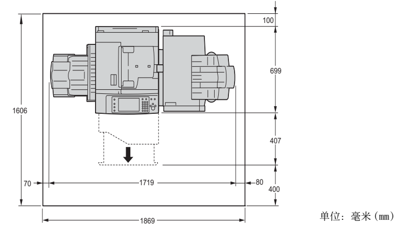
装有完成装订部 C3（选装）和侧接收盘（选装）时
