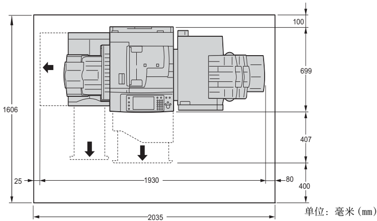
装有完成装订部 C3（选装）、侧接收盘（选装）和大容量纸盘 B1（选装）时
