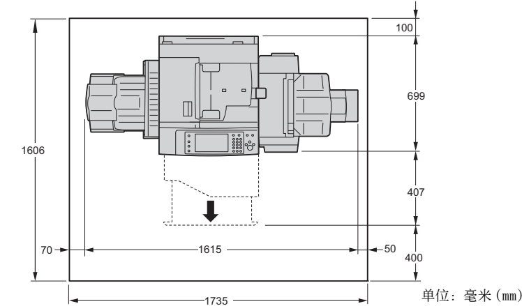
装有完成装订部 B1（选装）和侧接收盘（选装）时
