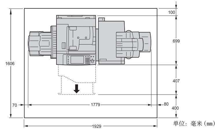
装有完成装订部 C3（小册子装订）（选装）和侧接收盘（选装）时
