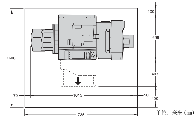
装有完成装订部 B1 用小册子装订组件（选装）和侧接收盘（选装）时
